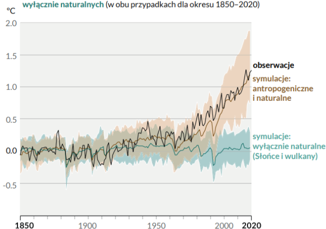
b) Zmiana globalnej temperatury powierzchni (średnie roczne): obserwowana i symulowana [modelami klimatu] przy uwzględnieniu czynników antropogenicznych i naturalnych oraz wyłącznie naturalnych (w obu przypadkach dla okresu 1850–2020)
