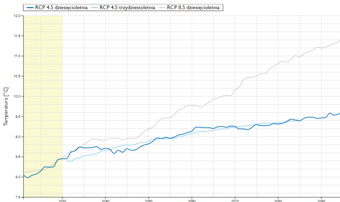
Ryc. 11 Scenariusz wzrostu średniej rocznej temperatury powietrza w powiecie giżyckim według scenariusza RCP 4.5 (wprowadzenie nowych technologii z redukcją emisji gazów cieplarnianych)
