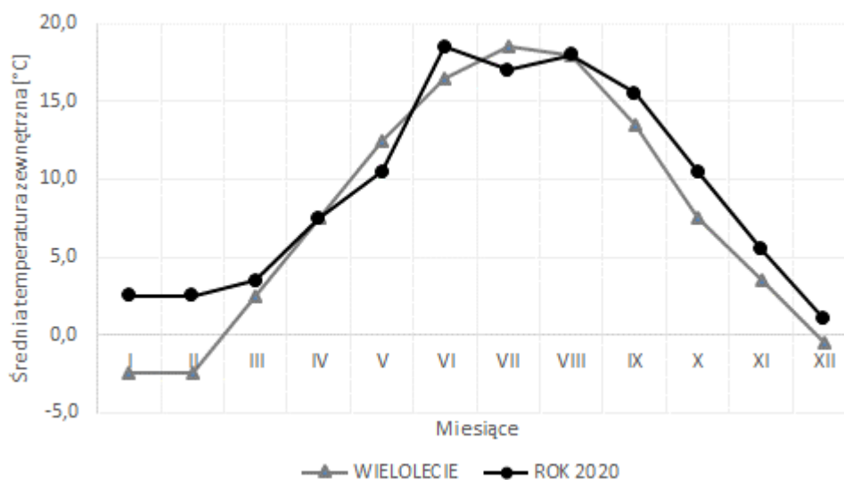
Ryc. 9 Rozkład średnich temperatur miesięcznych dla obszaru miasta Giżycka dla wielolecia 1991-2020 i 2020 roku
