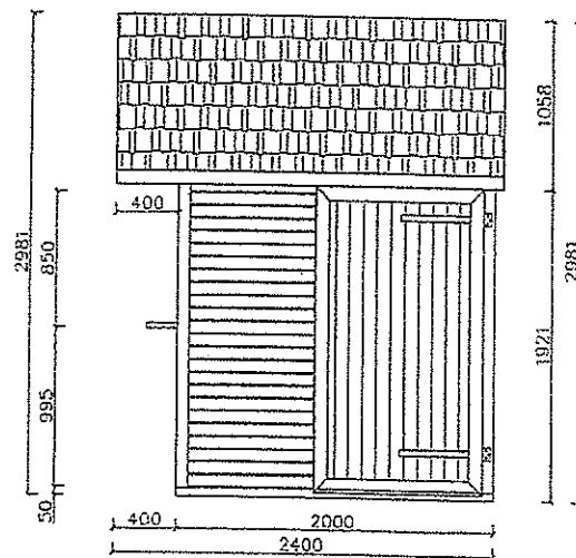
Elewacja boczna
