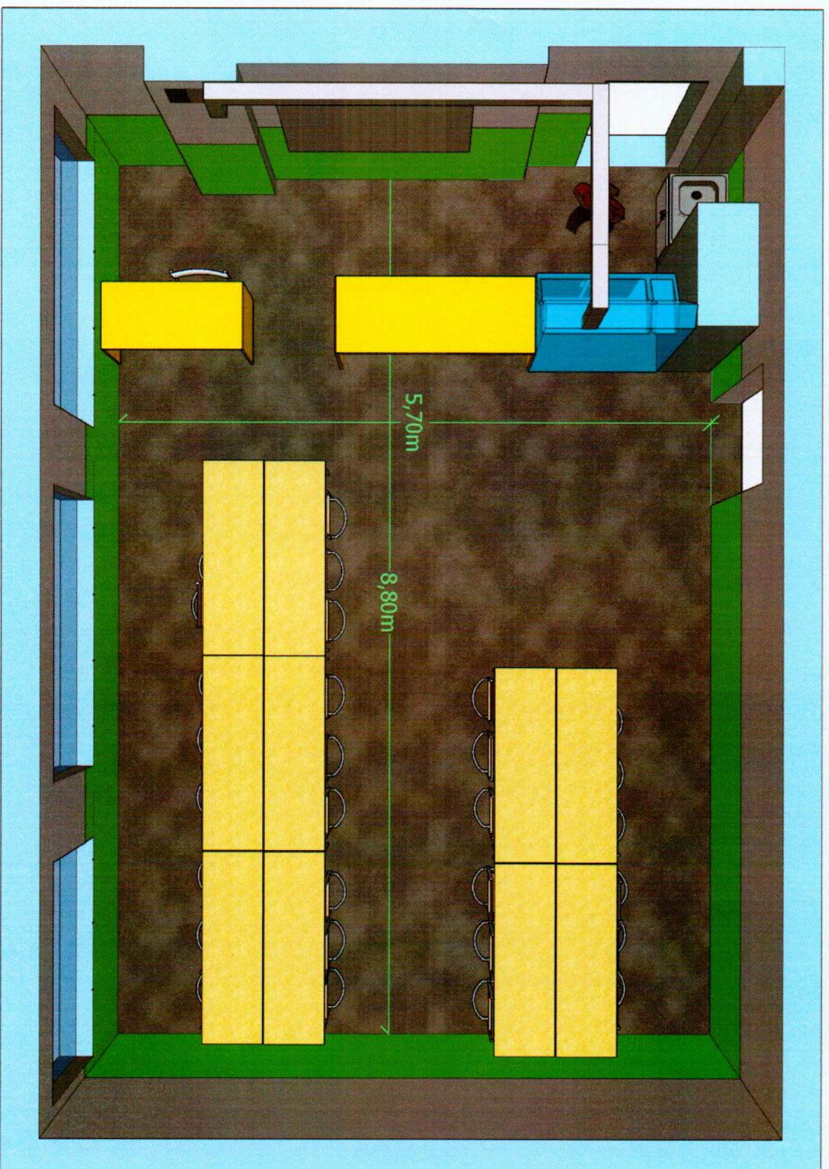
PLAN ROZMIESZCZENIA SPRZĘTÓW W KLASIE FIZYCZNO-CHEMICZNEJ W SZKOLE PODSTAWOWEJ NR 7 W GIŻYCKU
