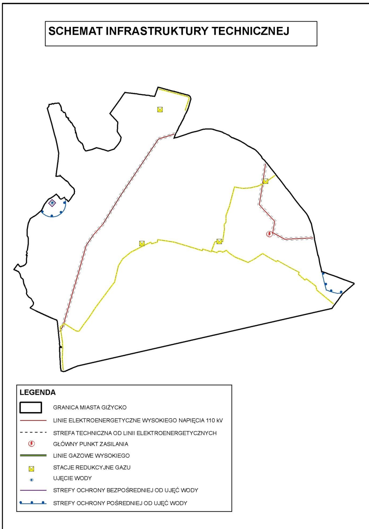
Ryc.41. Schemat infrastruktury technicznej na obszarze miasta Giżycko
