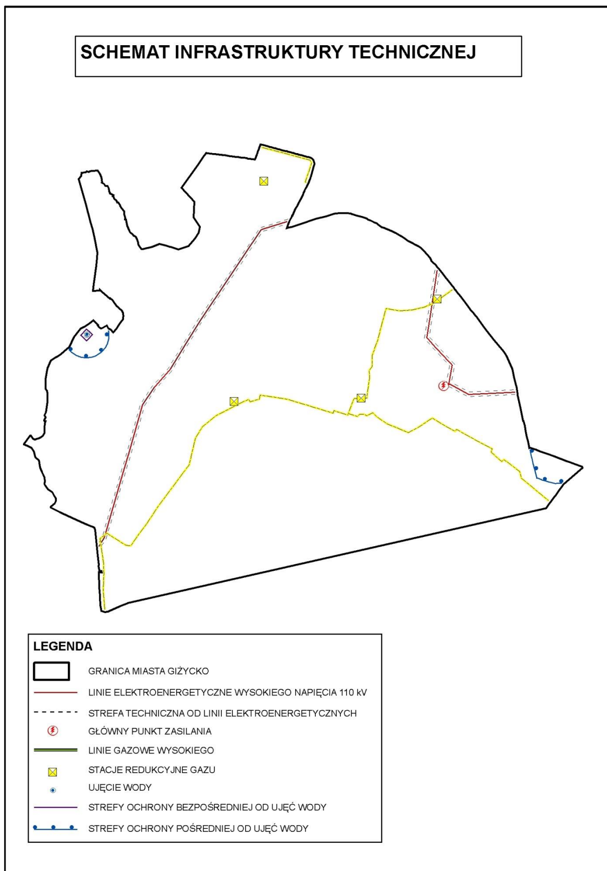
Ryc.40. Schemat infrastruktury technicznej na obszarze miasta Giżycko Źródło: Opracowanie własne
