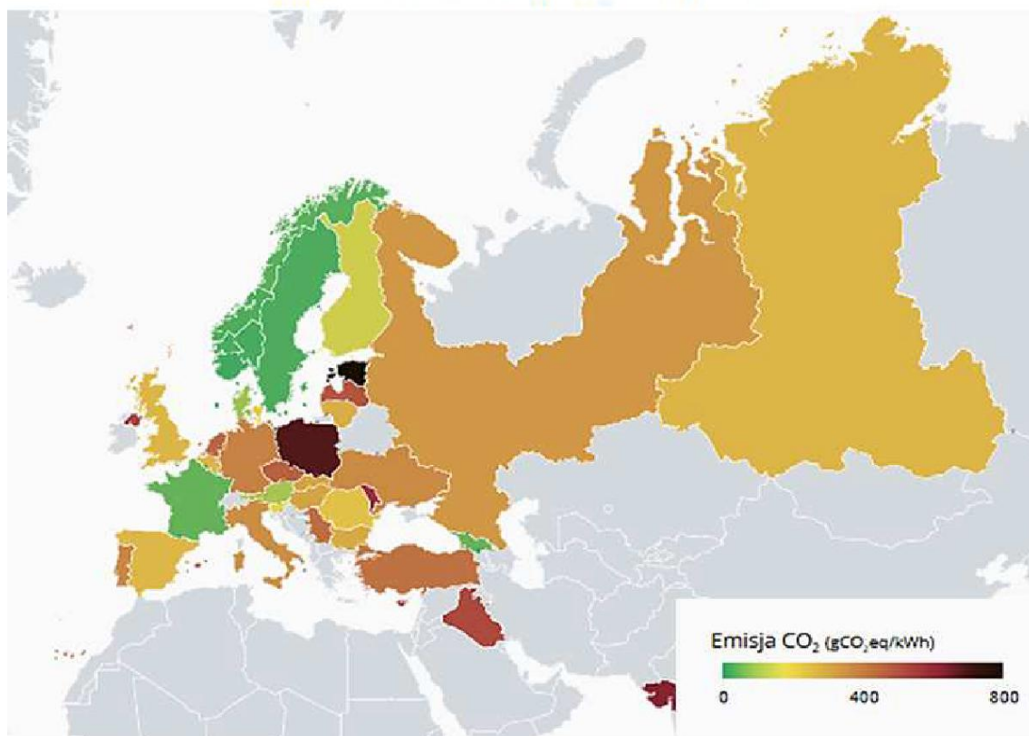
Rys.10 Emisja CO 2 na 1 kWh wyprodukowanej energii.
