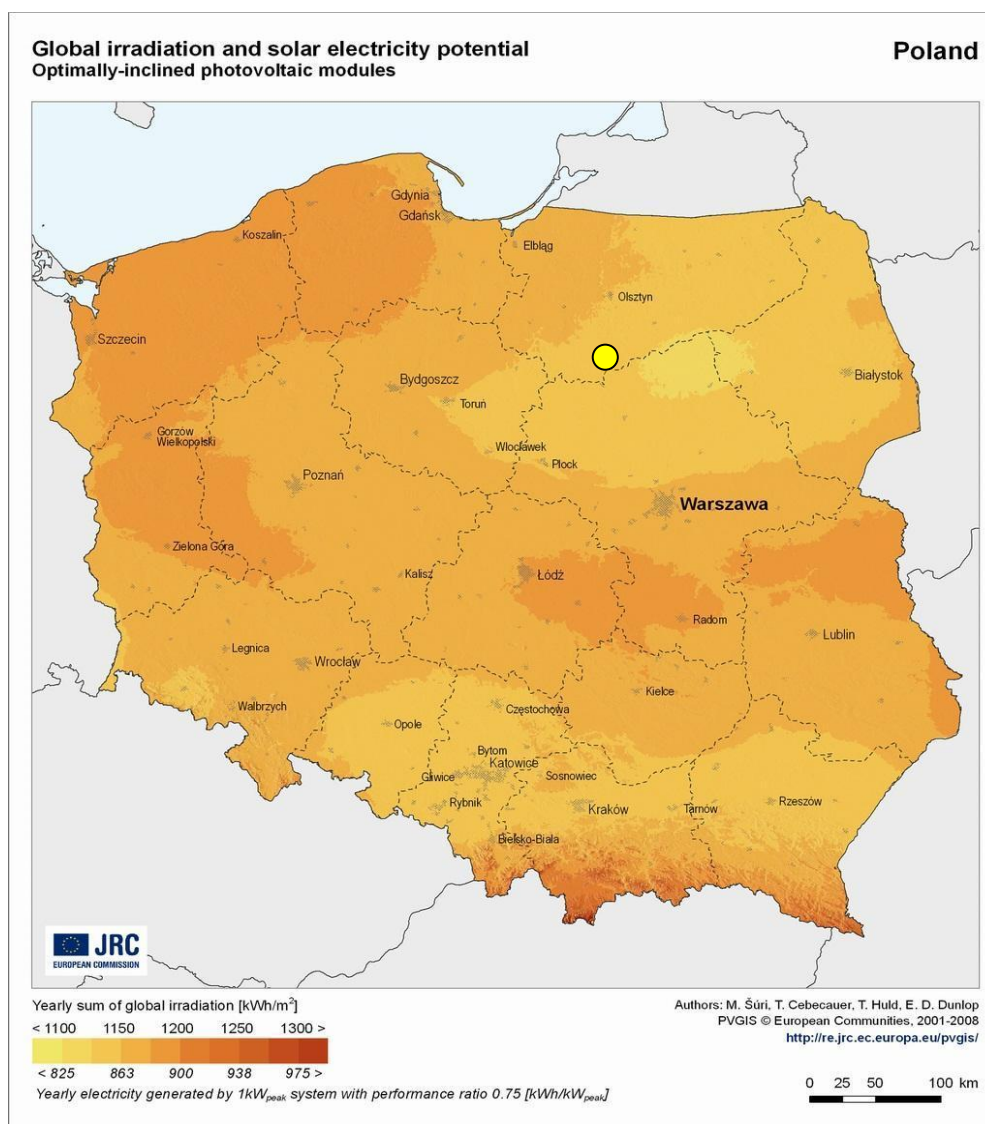
Rys.1 Klasyfikacja obszaru Polski pod względem nasłonecznienia.
