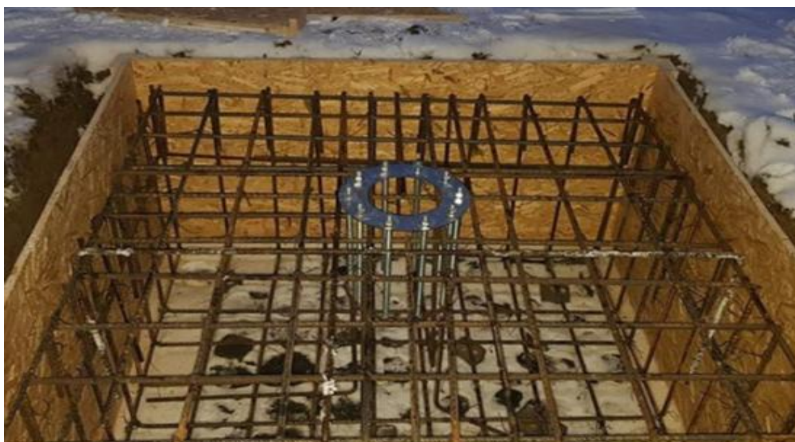
Rys.14 Fundamentowanie konstrukcji Trackera.
