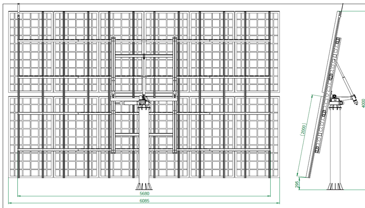
Rys.13 Parametry geometryczne Trackera.
