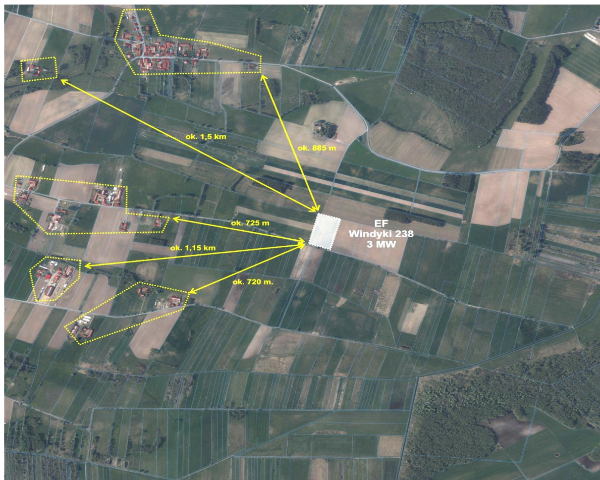
Rys.3 Lokalizacja planowanej elektrowni fotowoltaicznej w stosunku do najbliższej zabudowy mieszkalnej.
