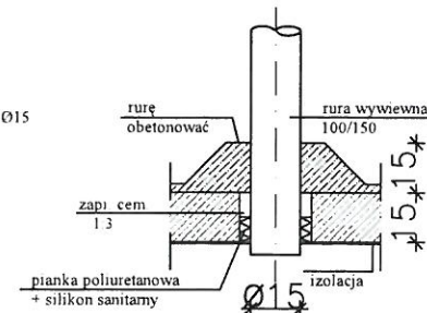
SZCZEGÓŁ "B"
