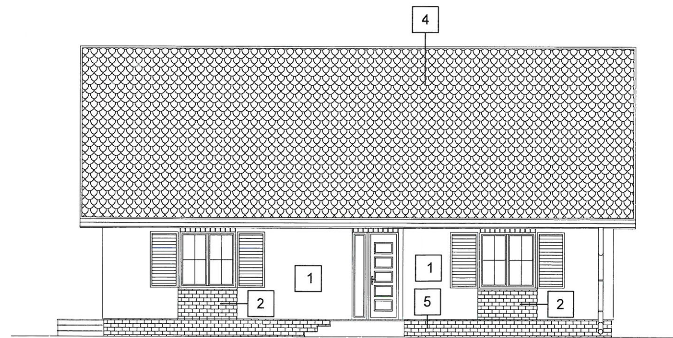
ELEWACJA POŁUDNIOWO - ZACHODNIA (TYLNA)
