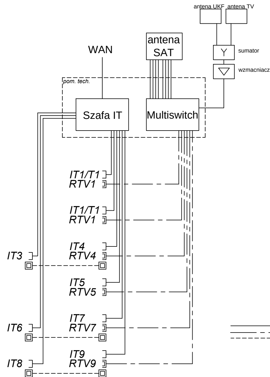
Schemat instalacji teletechnicznych
