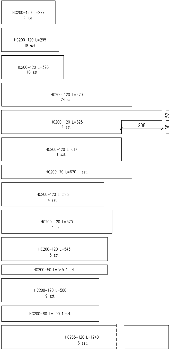
ZESTAWIENIE PÓŁ STROPOWYCH
