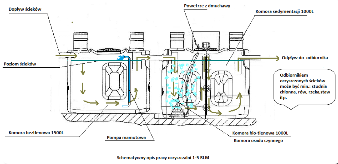
Rys. Przydomowa oczyszczalnia ścieków; Źródło: http://www.avitech.lap.pl/oczyszczalnie.html
