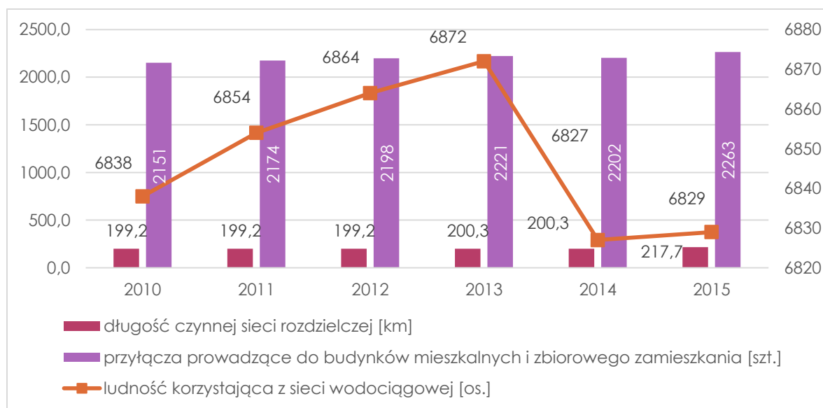
WYKRES 24 INFRASTRUKTURA WODOCIĄGOWA W GMINIE BODZANÓW W LATACH 2010-2015
