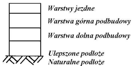
Rys. 4. Przykładowe wybrane konstrukcje nawierzchni utwardzonego pobocza z kruszywa łamanego niezwiązane
