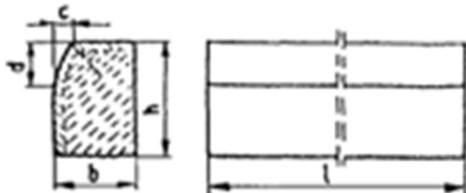
Rys. 2.1. Krawężnik betonowy typu ulicznego
